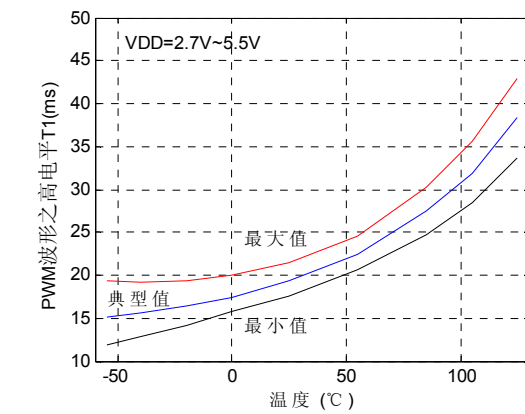
图 12. PWM 之高电平时间
