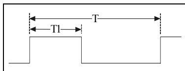
图 3. PWM 波形图
