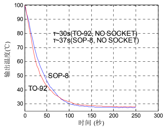
图 8. 温度响应时间
