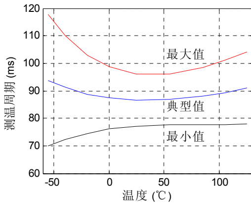
图 9. 测温周期
