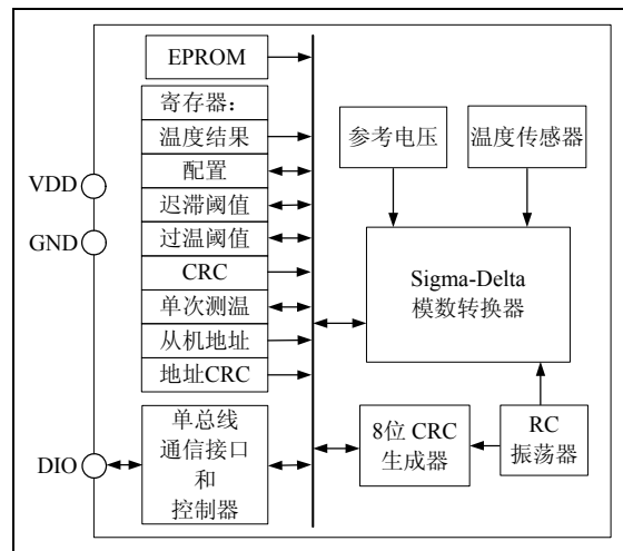
图 2. 功能框图
