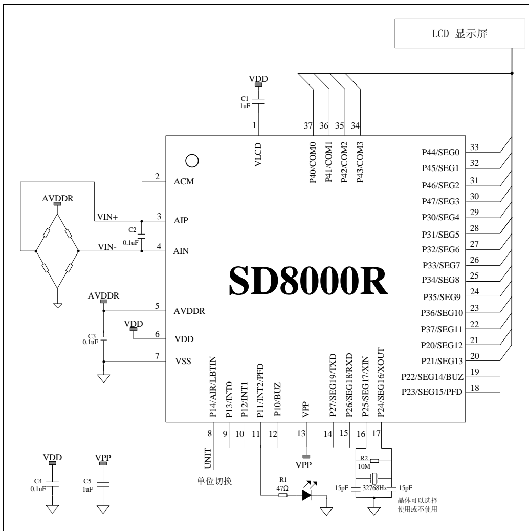
图 3. 带时钟的 LCD 显示人体秤典型应用图
