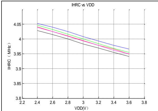
图 4. IHRC 电压特性曲线
