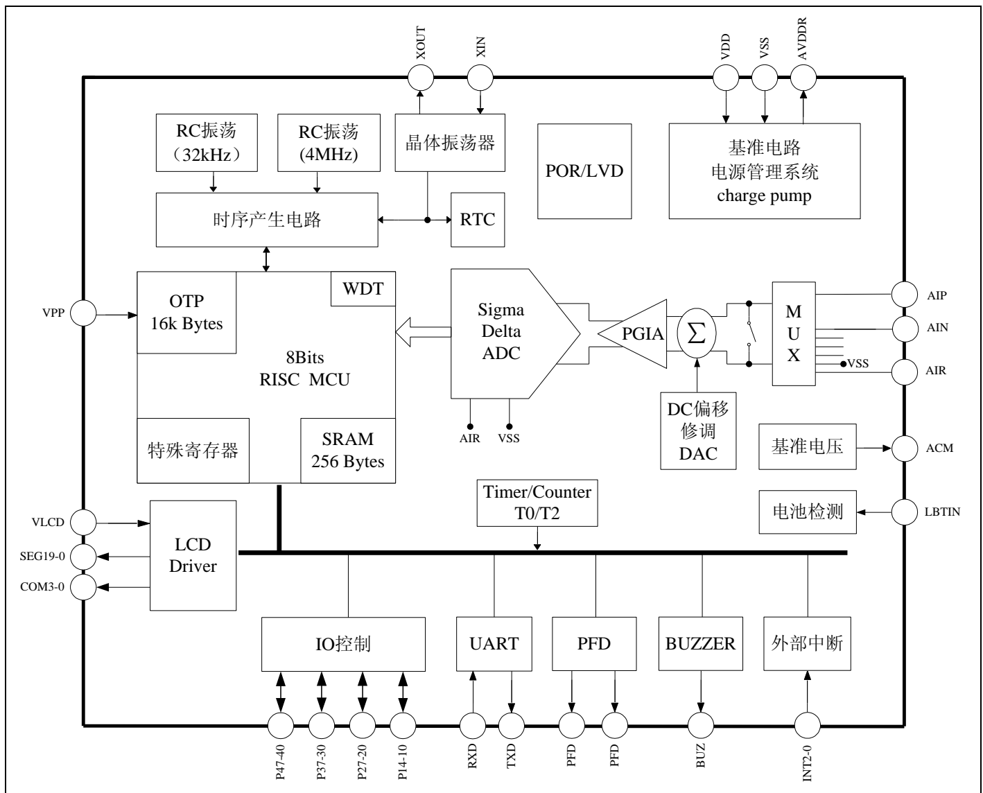
图 2. 功能框图
