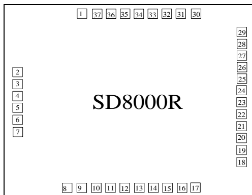
图 1. PAD 图
